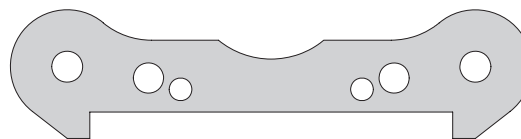
86070 Lower Arm Brace 4x54x3mm Untere querlenkerstrebe 4x54x3mm Support bras inferieur 4x54x3mm ロアアームブレース 4x54x3mm
