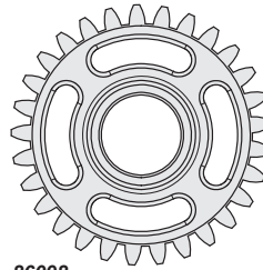
86098 Idler Gear 29 Tooth Getriebezahnrad 29 Zahne Pignon intermediaire 29 Dents アイドルギヤ 29T
