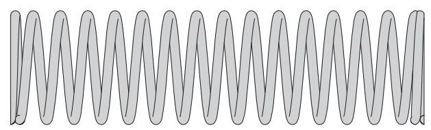
86551 Shock Spring 18x80x1.8mm 14.5 Coils (Pink 134gf/mm) Daempferfeder 18x80x1.8mm 14.5 Wdg (Pink 134gf/mm) Ressort Am. 18x80x1.8mm 14.5 Sp. (Rose 134gf/mm) ショックスプリング 18x80x1.8mm 14.5巻 (ピンク 134gf/mm)
